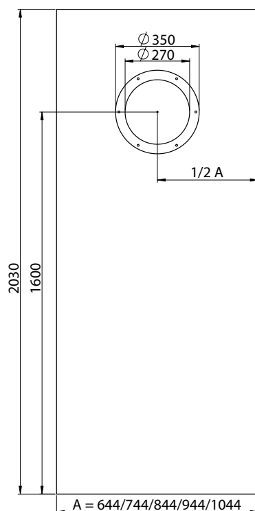
Budowa skrzydła Bulaj przylgowego
