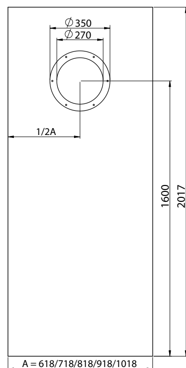
Budowa skrzydła Bulaj bezprzylgowego
